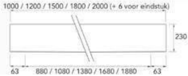
Standaard eindstuk
